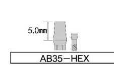
HEX嵌合アングラアバットメント(AG35-D05のみグループ付) Bタイプと共通
