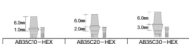
HEX嵌合ストレートアバットメント(グループ無) Cタイプと共通
