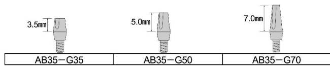
テーパー嵌合ストレートアバットメント(グループ付) Bタイプと共通
