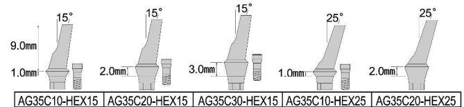
HEX嵌合アングラアバットメント(グループ付) Cタイプと共通
