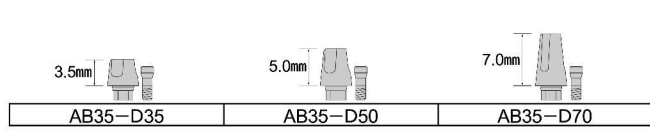
テーパー嵌合アングラアバットメント Bタイプと共通
