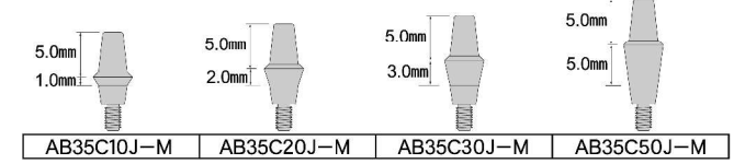
テーパー嵌合ストレートアバットメント(グループ無) Cタイプと共通
