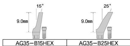
HEX嵌合アングラアバットメント(グループ無) Bタイプと共通
