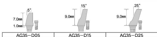
HEX嵌合アングラアバットメント(AG35C-D05のみグループ付) Cタイプと共通
