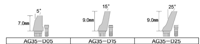
HEX嵌合アングラアバットメント(AG35-D05のみグループ付) Bタイプと共通
