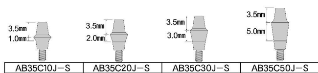
テーパー嵌合ストレートアバットメント(グループ無) Cタイプと共通
