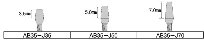
テーパー嵌合ストレートアバットメント(グループ無) Bタイプと共通
