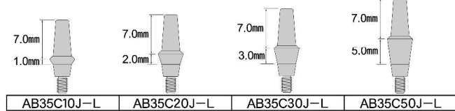
テーパー嵌合ストレートアバットメント(グループ無) Cタイプと共通
